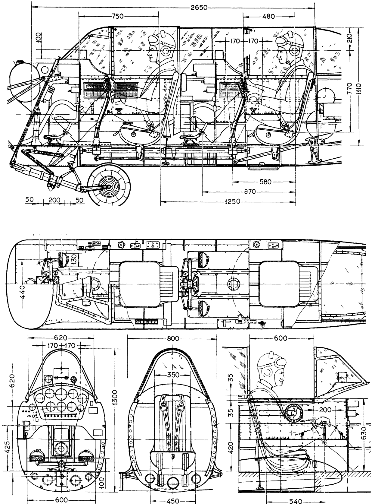
Рис. 2 Компоновка кабины
