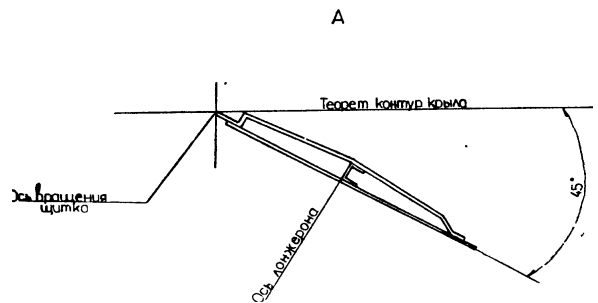
Рис. 8 Схема щитка
