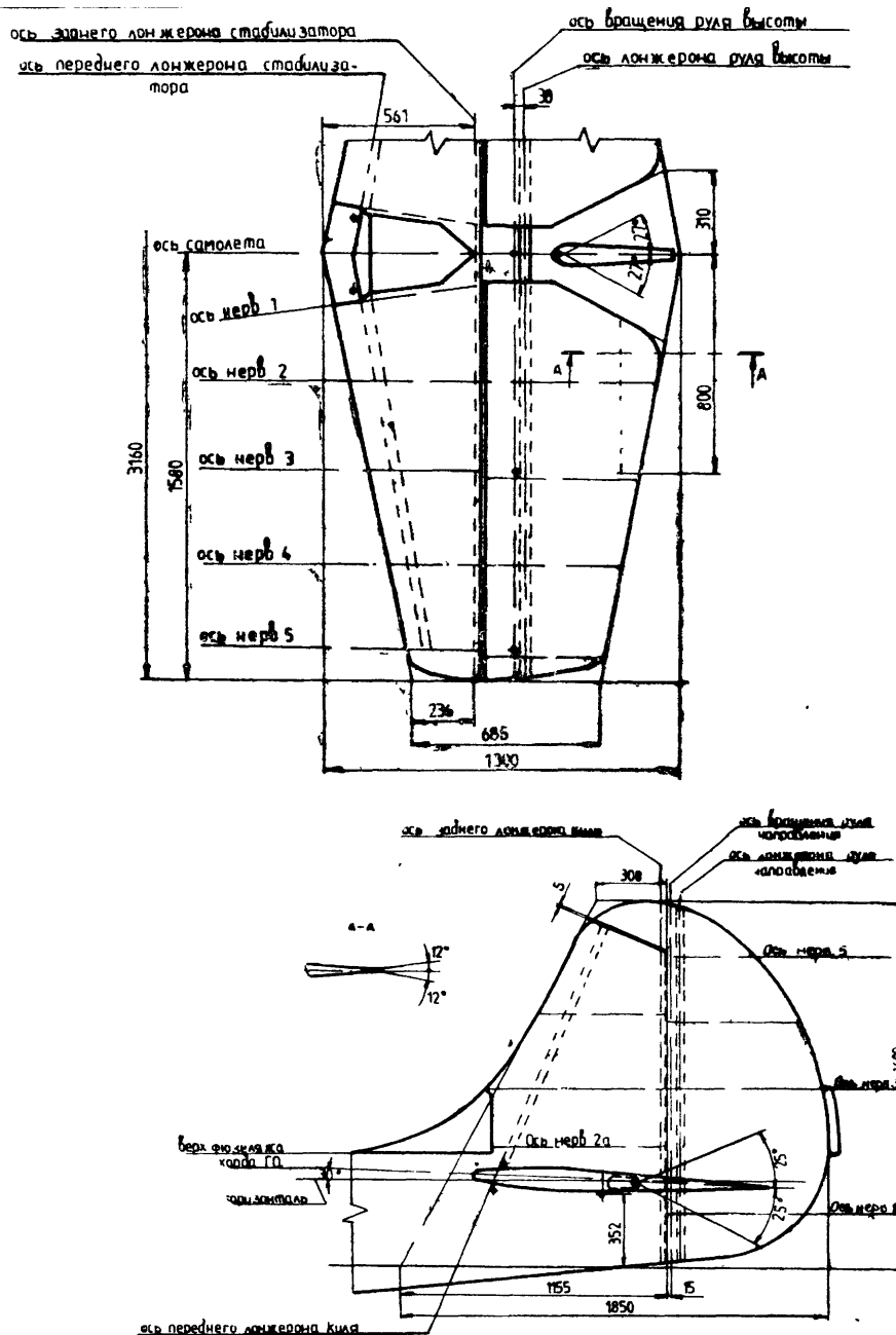
Рис. 10 Схема оперения
