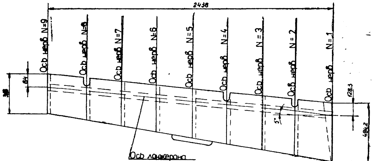
Рис. 6 Схема элерона
