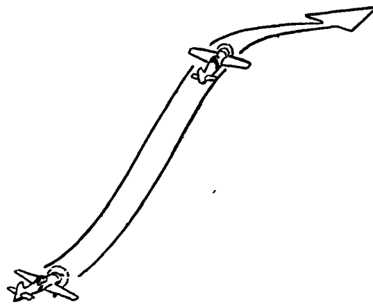
Горка
