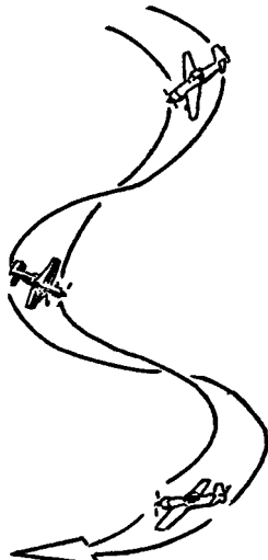
Штопор
