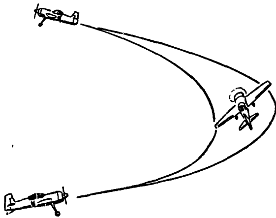
Боевой разворот
