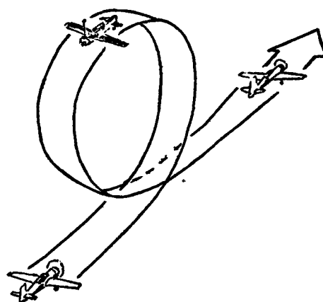
Петля Нестерова
