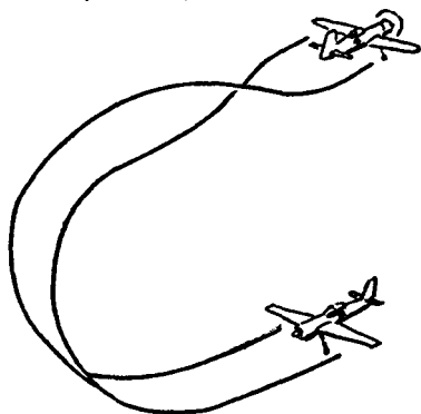
Полупетля
