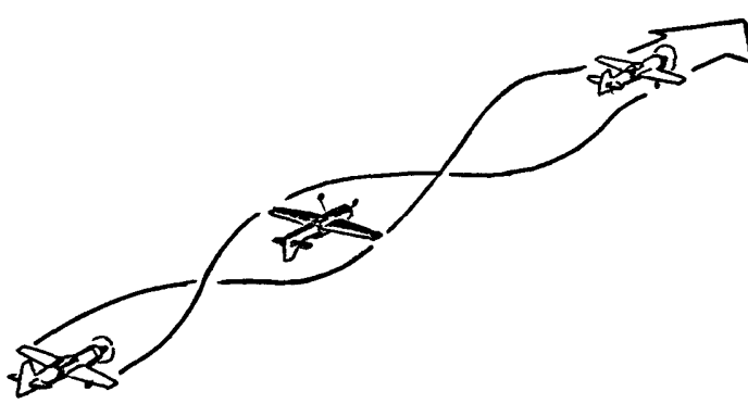
Бочка
