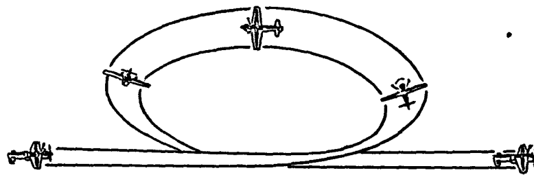
Обратный вирах
