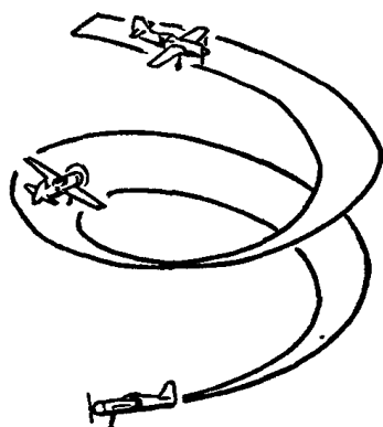
Спираль
