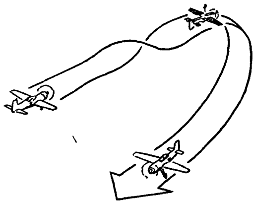
Переворот
