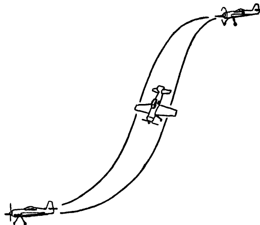
Пикирование
