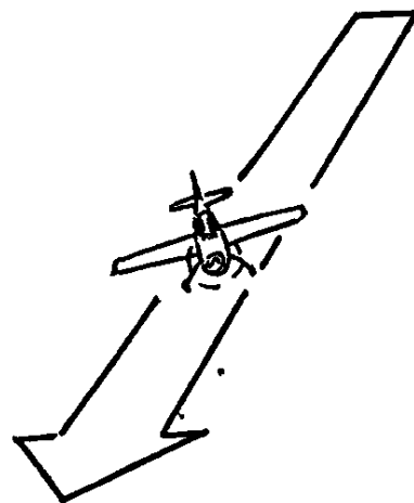
Скольжение
