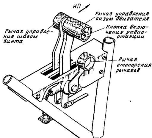
Рычаги управления двигателем.
