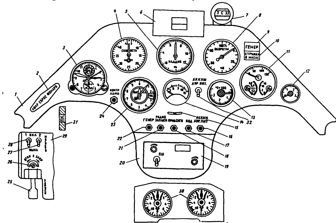
Размещение оборудования в кабине
