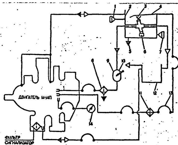
Масляная система
