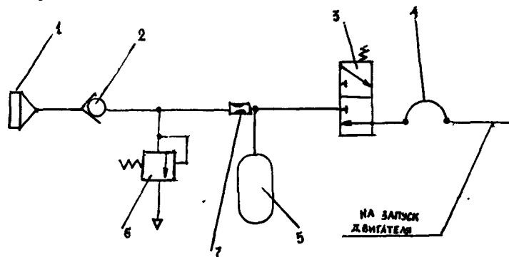
Пневматическая система самолета.
