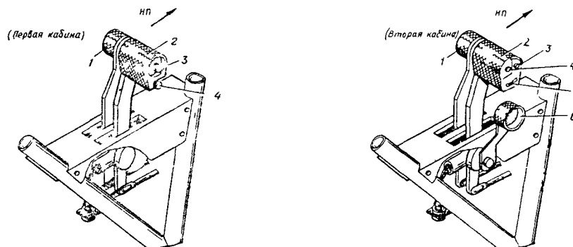
Рис 5. Рычаг управления двигателем и шагом винта
