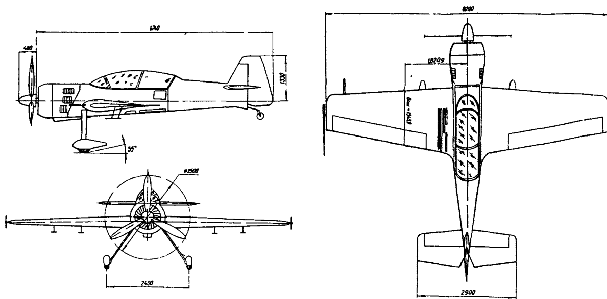
Рис. 1. Общий вид самолета
