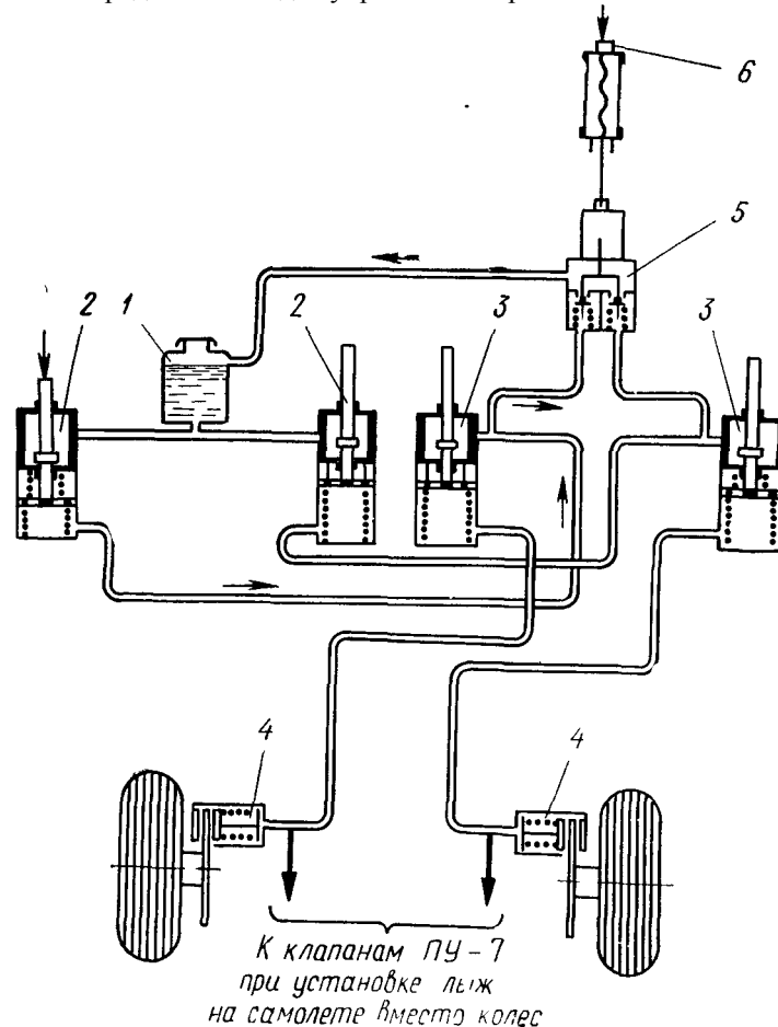
Рис. 7. Схема гидросистемы
