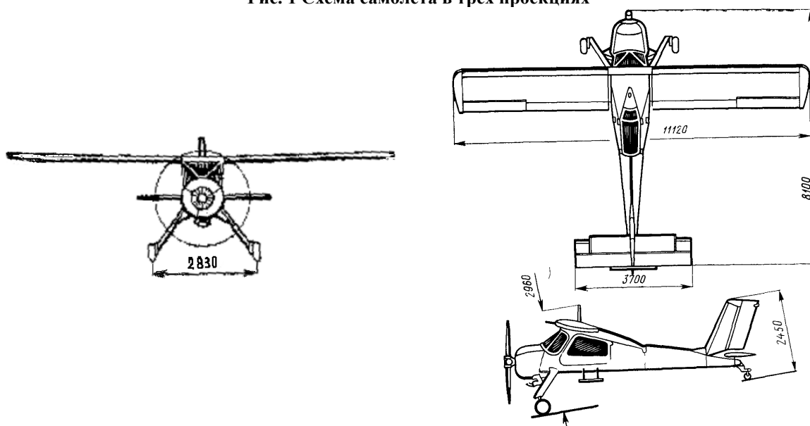
Рис. 1 Схема самолета в трех проекциях
