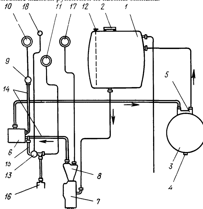
Рис. 10. Схема масляной системы
