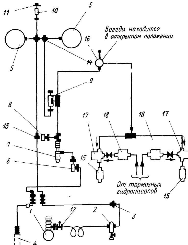
Рис 8. Схема воздушной системы
