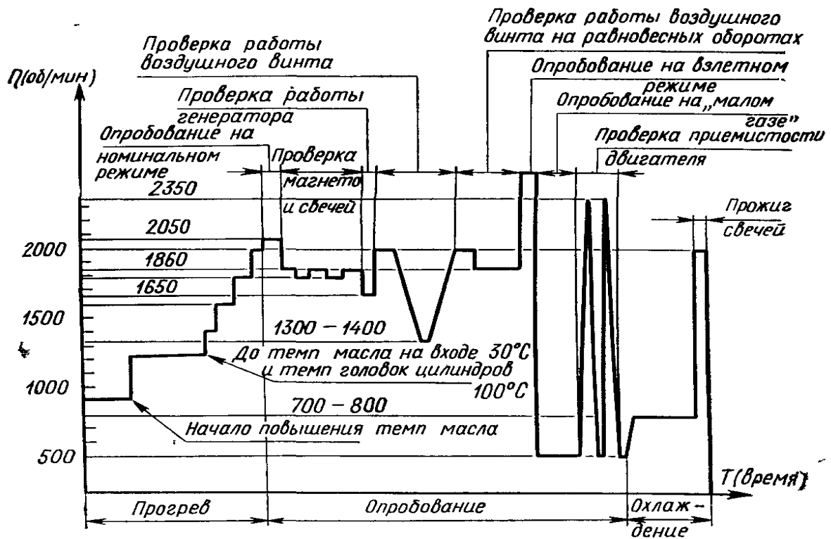
Рис. 5. График опробования двигателя
