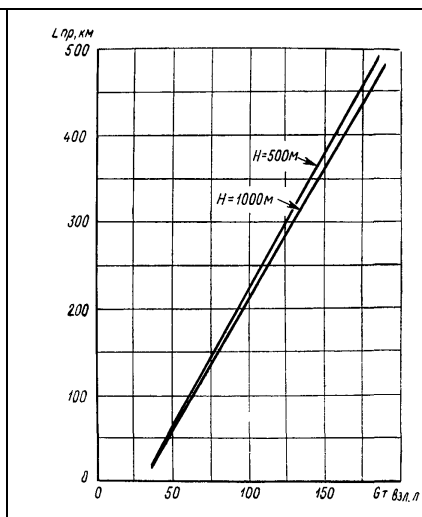
Рис. 3. Дальность полета самолета с лыжным шасси в зависимости от запаса топлива при взлете и высоты полета
