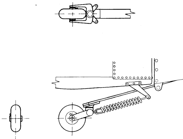
Хвостовая опора с амортизатором
