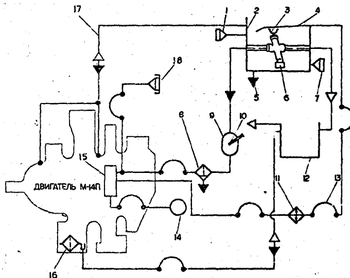
Рис. 6.2. МАСЛЯНАЯ СИСТЕМА.
