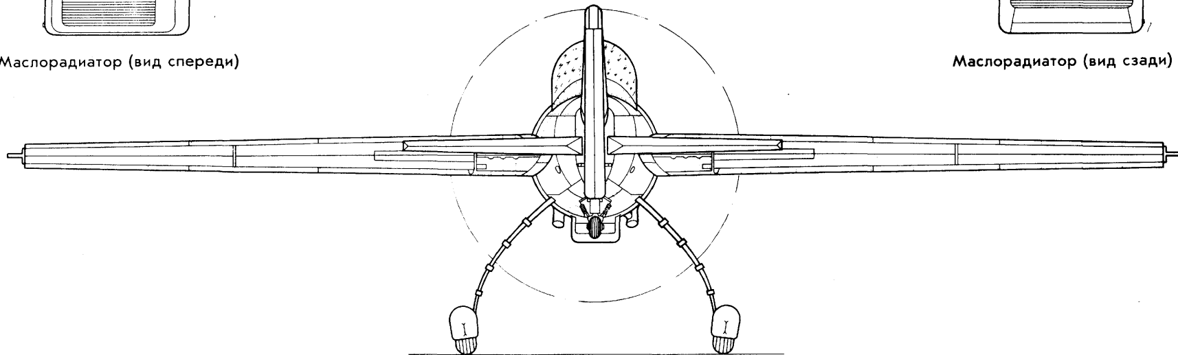
ЯК-55 (вид сзади)
