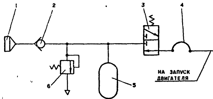
Рис. 6.3. ВОЗДУШНАЯ СИСТЕМА
