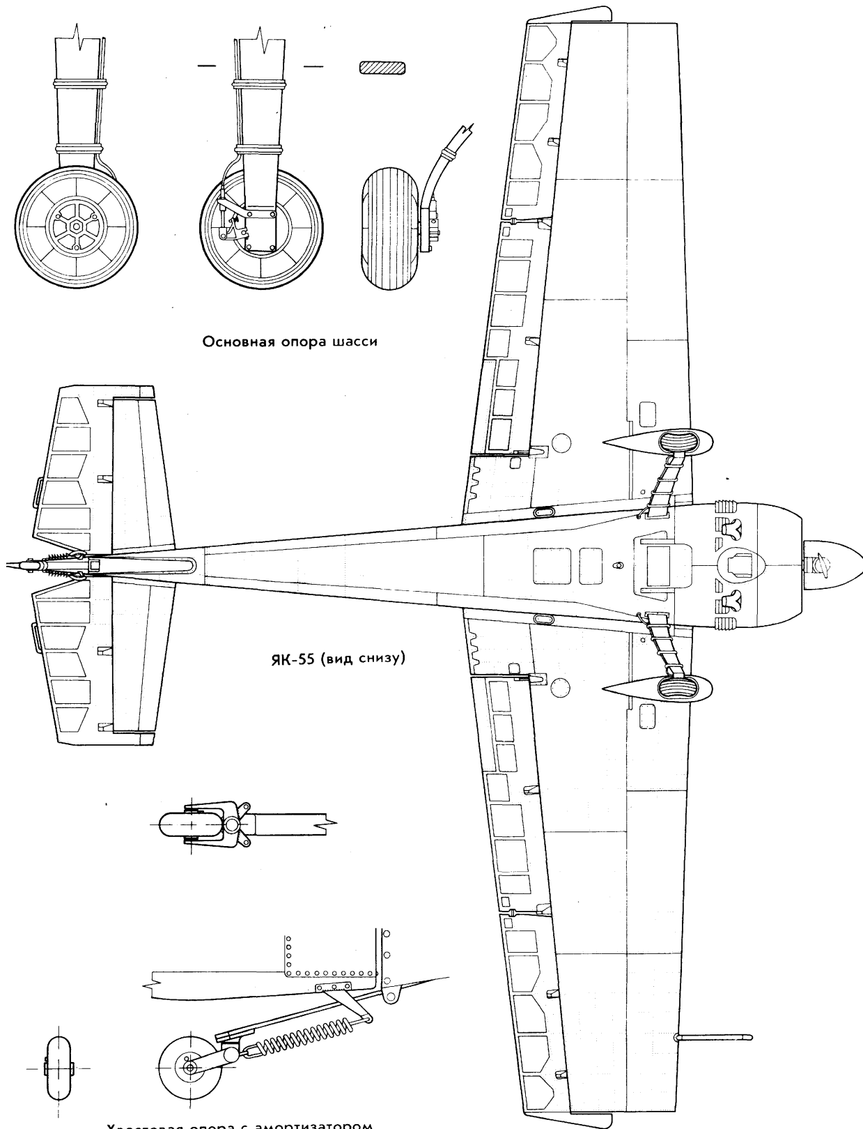
Хвостовая опора с амортизатором
