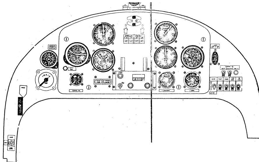
Рис. 6 Приборная доска самолета Як-55.
