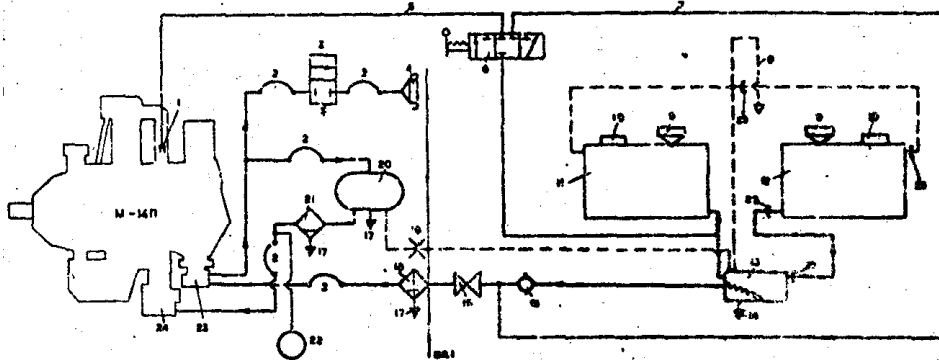
Рис. 6.1. ТОПЛИВНАЯ СИСТЕМА
