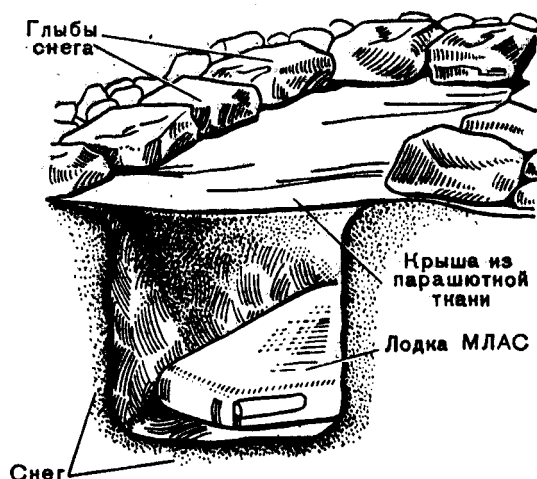
Рис. 10 Постройка снежной траншеи
