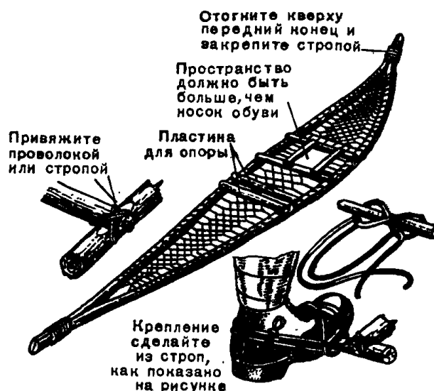
Рис. 28 Изготовление лыж-снегоступов из подручных средств
