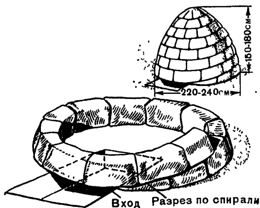
Рис. 12 Постройка снежной хижины типа «иглу»
